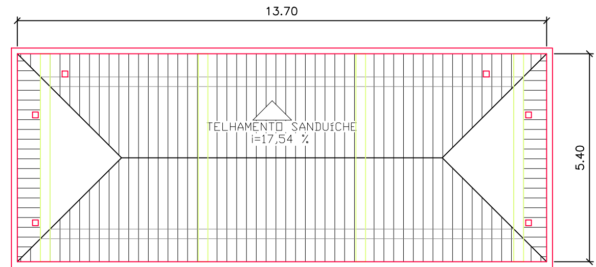
PLANTA DE COBERTURA Esc 1/100
