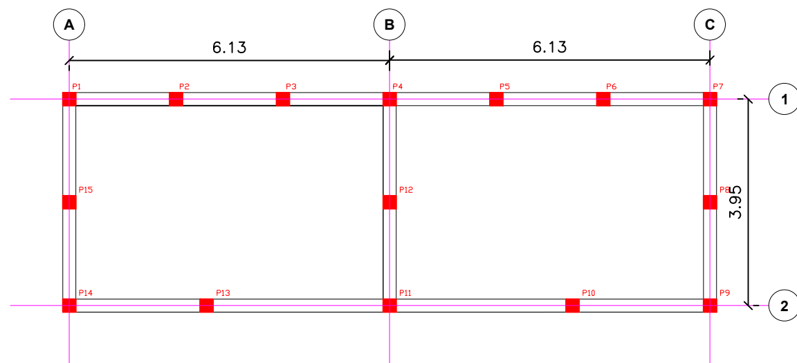
PLANTA DE MARCAÇÃO Esc 1/100
