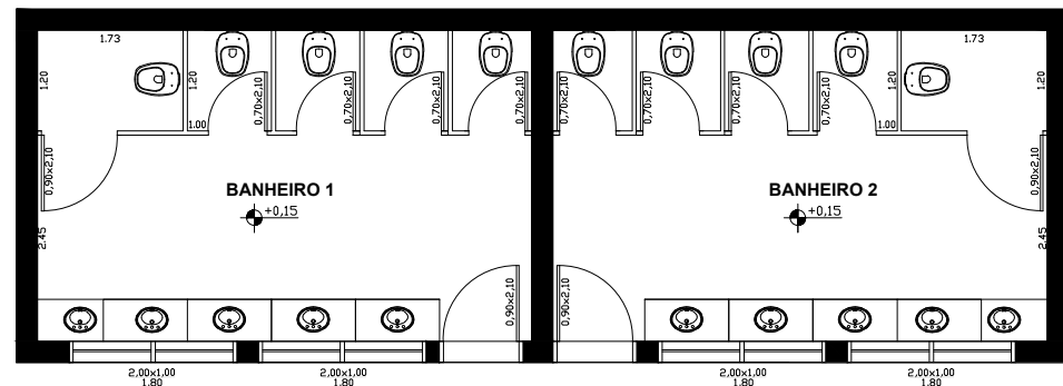
PLANTA BAIXA BANHEIRO FEMININO E MASCULINO Esc 1/100
