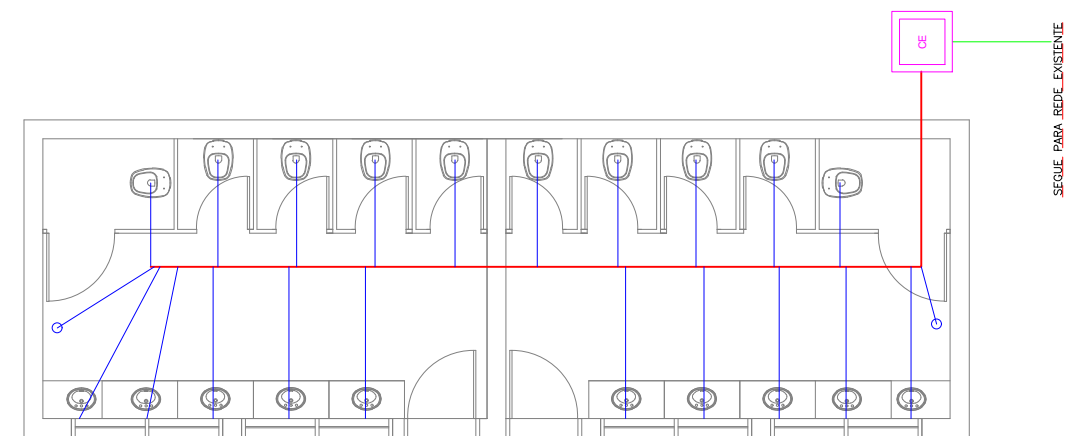
PLANTA DE HIDRÁULICA Esc 1/100
