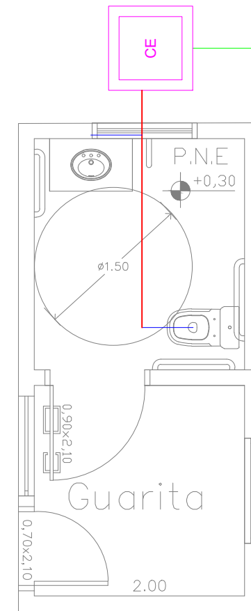
PLANTA HIDRÁULICA Esc 1/50
