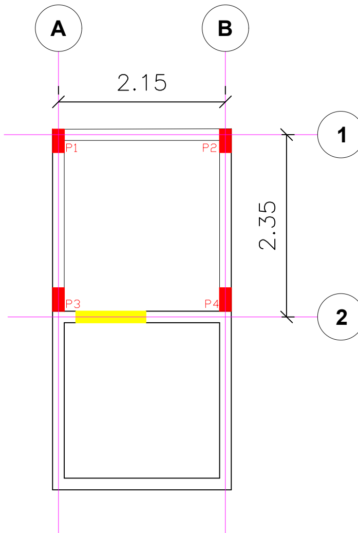
PLANTA DE MARCAÇÃO Esc 1/50
