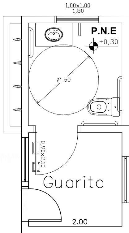
PLANTA BAIXA GUARITA RUA 14 E RUA 10 Esc 1/50
