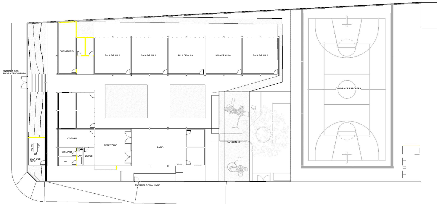
1 PLANTA BAIXA - DEMOLIÇÃO 1:100
