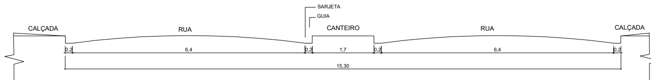
02. CORTE TRANSVERSAL A-A DAS RUAS ESC: 1/100
