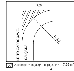
05. DETALHE DA EXTREMIDADE DO CANTEIRO ESC: 1/50
