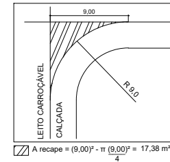
04. DETALHE DO RAIO ESC: 1/10 Detalhe avenida N
