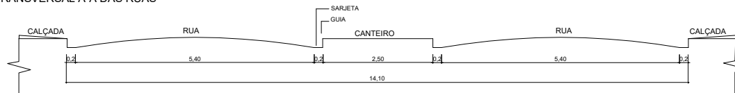
02. CORTE TRANSVERSAL A-A DAS RUAS ESC: 1/100
