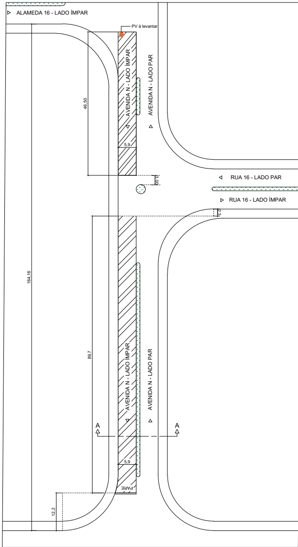
01. PLANTA DE SITUAÇÃO ESC: 1/1000
