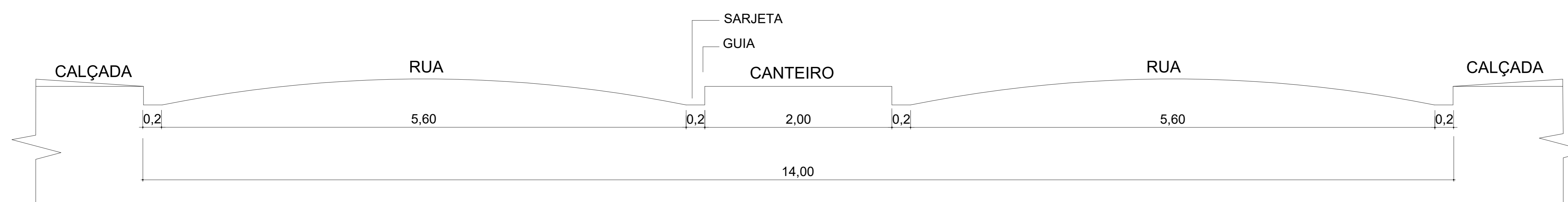
02. CORTE TRANSVERSAL A-A DAS RUAS ESC: 1/100
