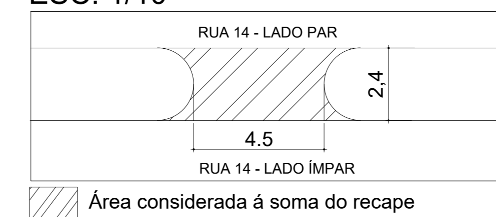
06. DETALHE MEIO DO CANTEIRO ESC: 1/10
