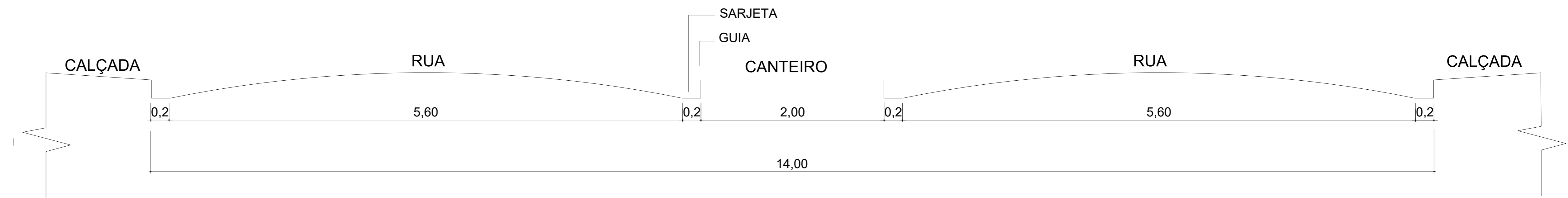
02. CORTE TRANSVERSAL A-A DAS RUAS ESC: 1/100
