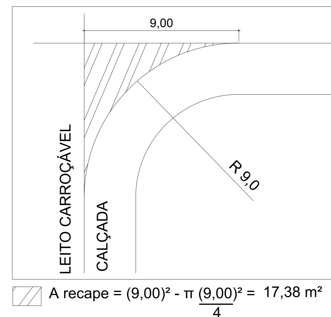
04. DETALHE DO RAIO ESC: 1/10 Detalhe rua 14
