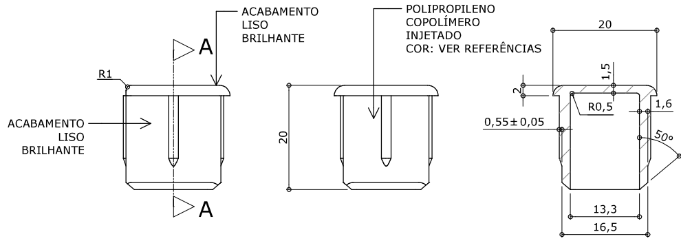
VISTA 1 ESC. 1 : 1
