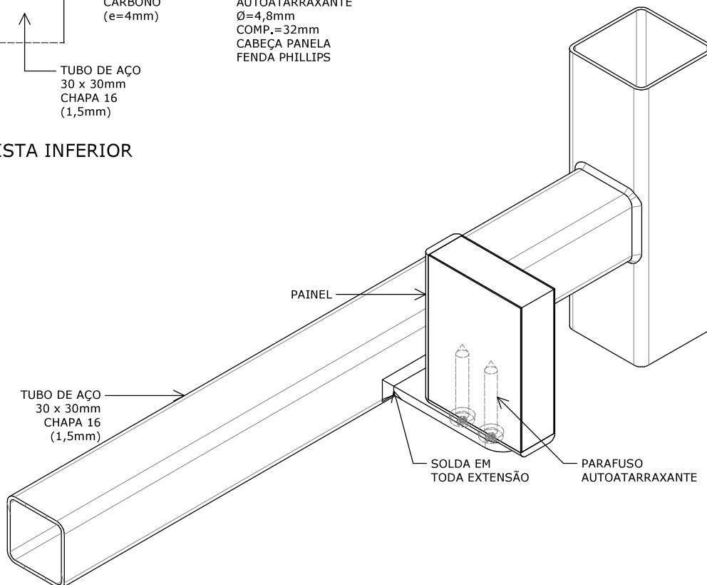
DETALHE 2
